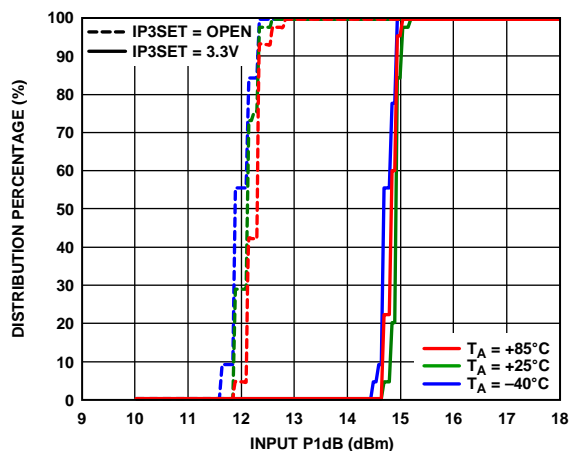
Figure 30. Input P1dB
