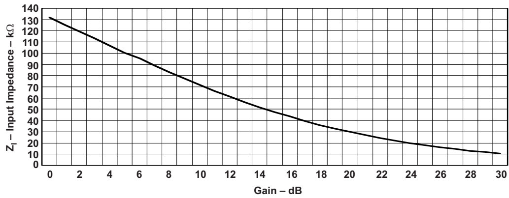
Figure 28. Nominal Input Impedance - Per Leg
