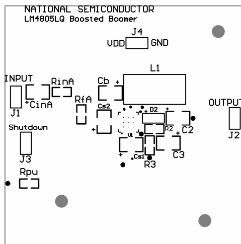
Figure 47. Bottom Layer
