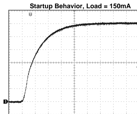
CH1: V_{OUT} ; Scale: 200mV/Div, DC Coupled Time scale: 20µs/Div
